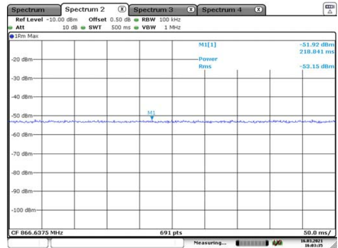
867.1-0,5 x OCW - 400 kHz
